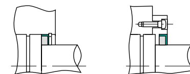
图E-8 毛毡密封环的安装范例
